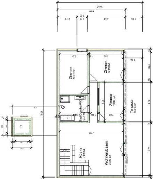
Erdgeschoss
